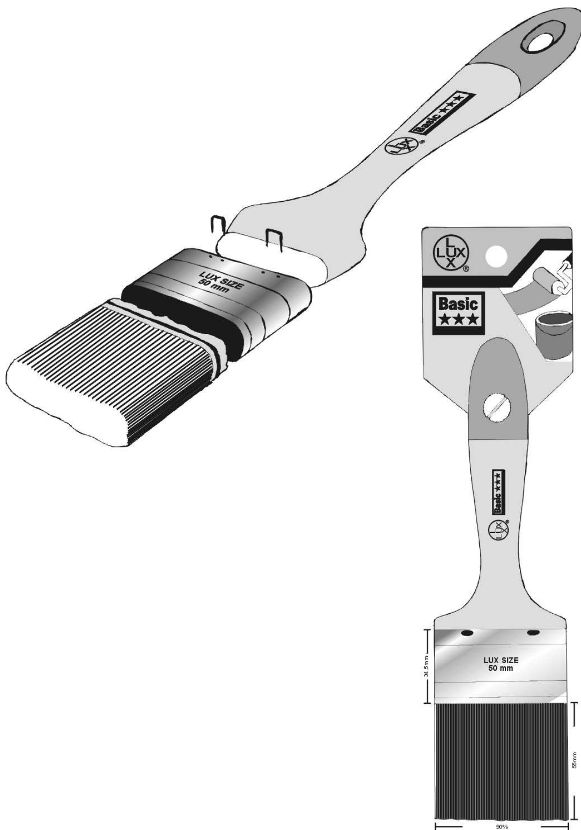
FIGURA 17 – Pincel LUX
