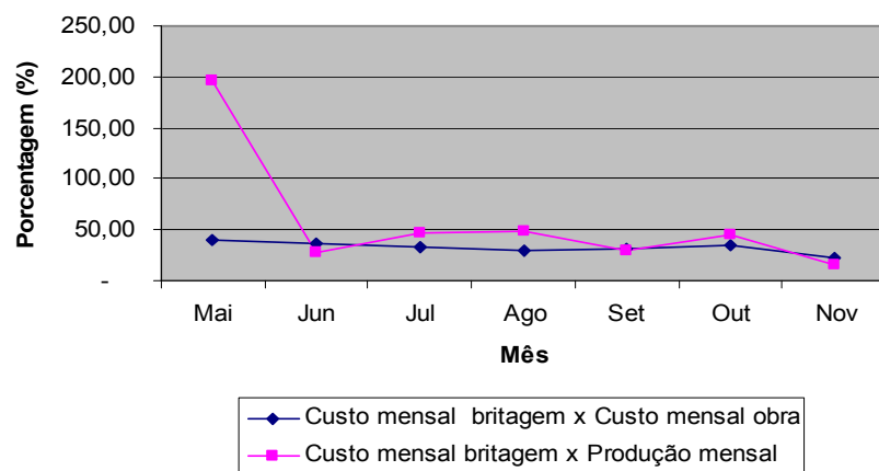
Figura 24 Gráfico Custo Mensal Britagem versus Custo Mensal Obra versus Produção Mensal (percentuais) Fonte: Relatórios mensais da empresa (2005).
