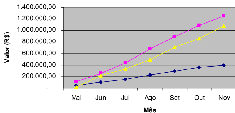
Figura 22 Gráfico Custo Mensal Britagem versus Custo Mensal Obra versus Produção Mensal Obra(2005) Fonte: Relatórios mensais da empresa (2005)
