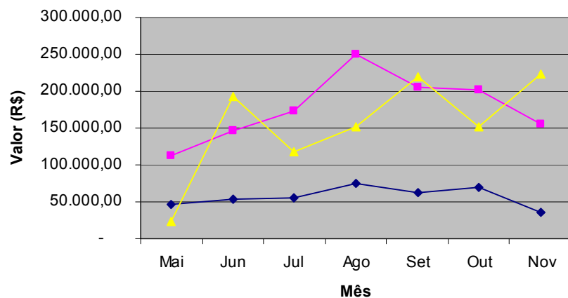
Figura 22 Gráfico Custo Mensal Britagem versus Custo Mensal Obra versus Produção Mensal Obra(2005) Fonte: Relatórios mensais da empresa (2005)
