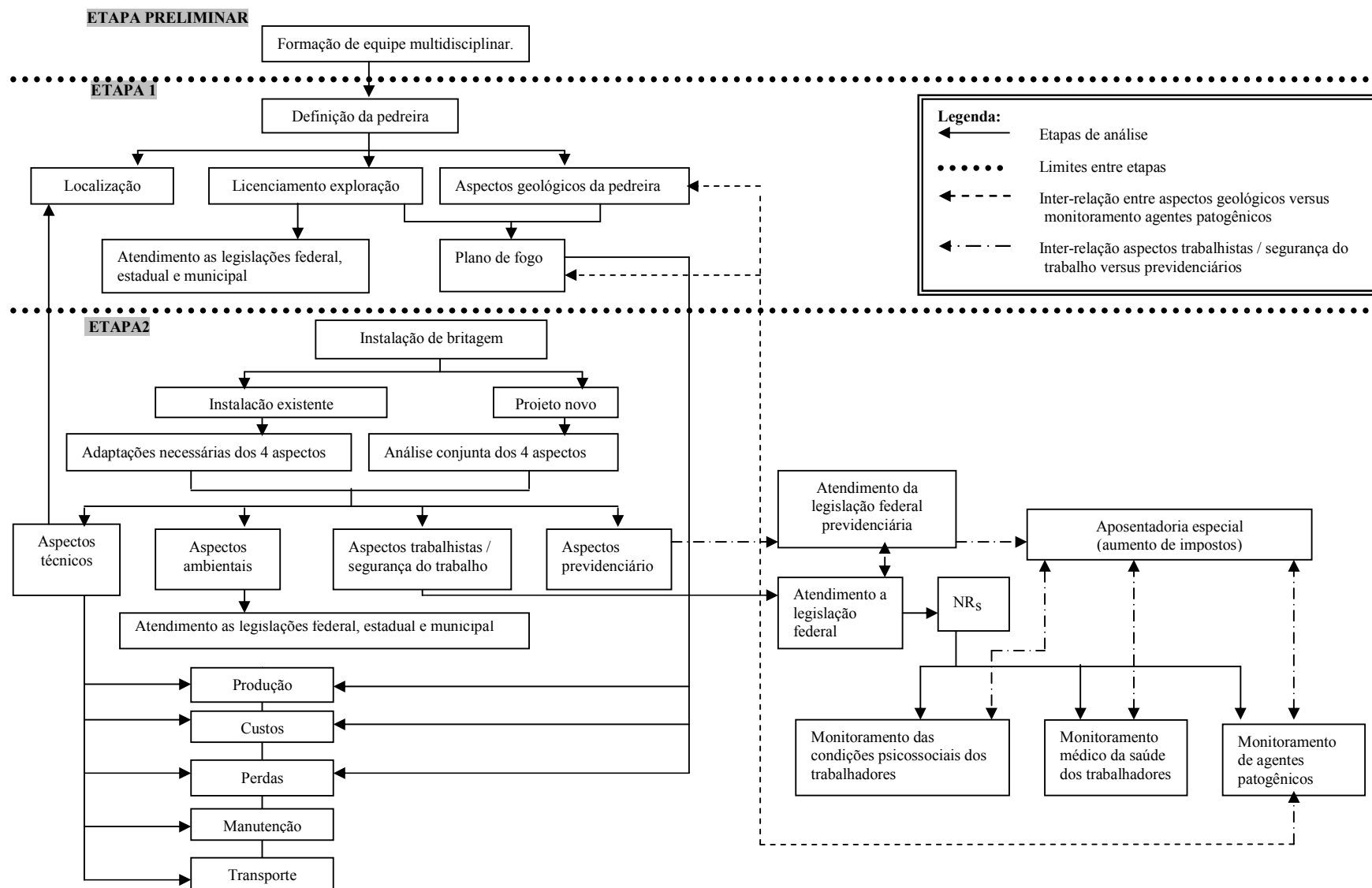
Figura 63 Modelo para Análise de Instalações de Britagem
