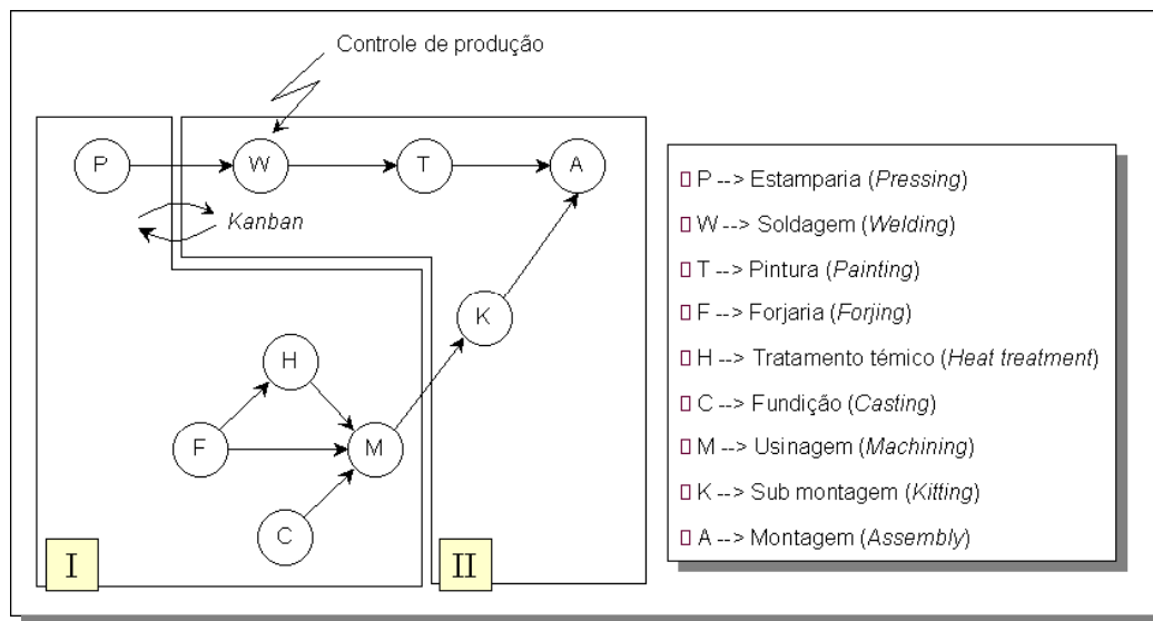
Figura 1 – Representação esquemática do processo de fabricação automobilístico (Adaptado de Toyota Motor Company, 1998).
