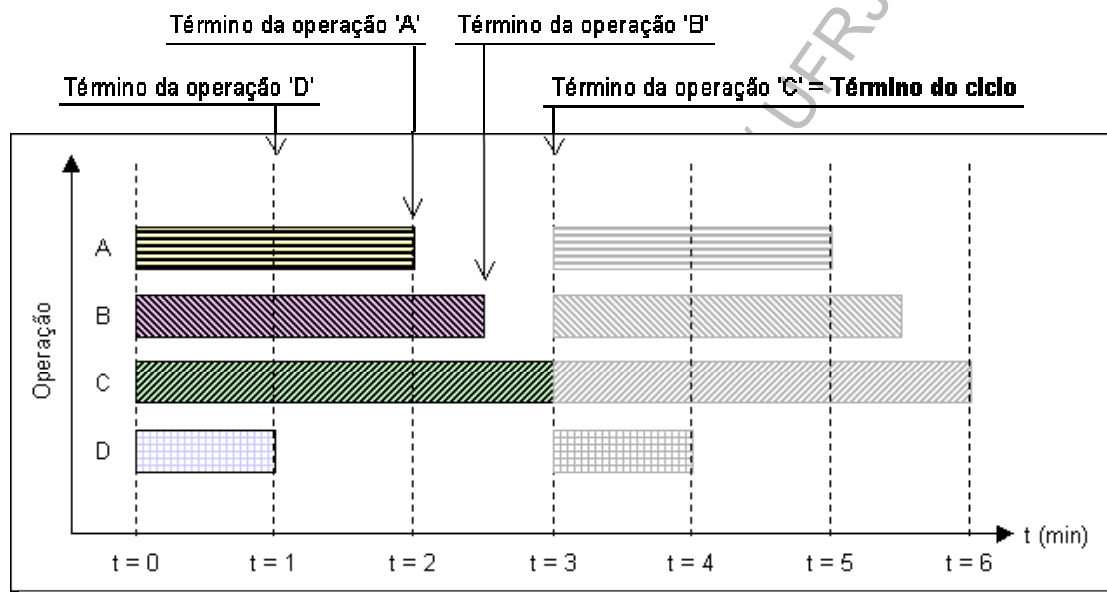
Figura 3 – Tempo de ciclo para o exemplo da Figura 2
